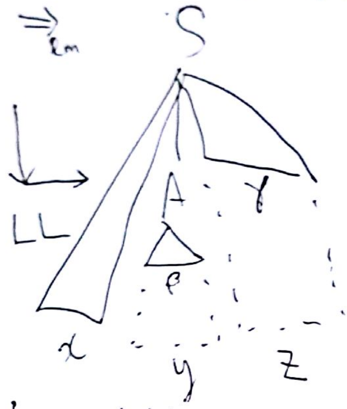
Lemma 4.6(Ext)
